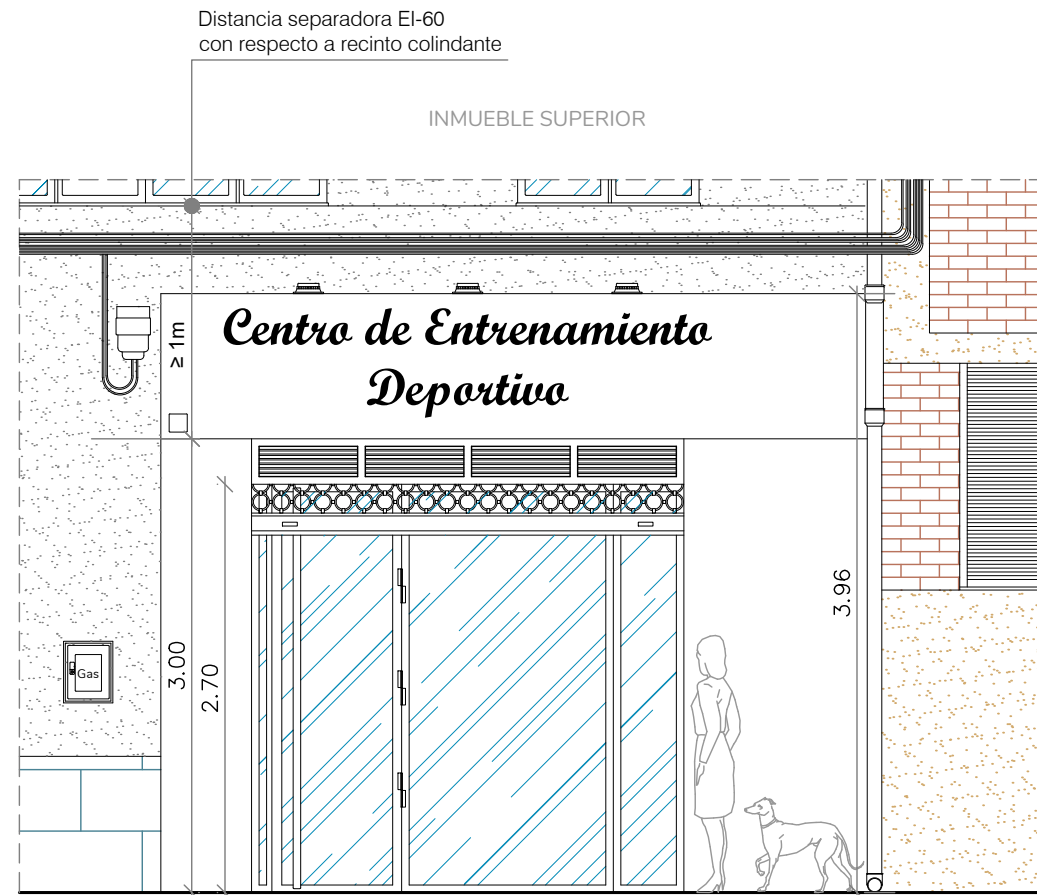
ALZADO EN ESTADO PROPUESTO DE FACHADA E:1/50
