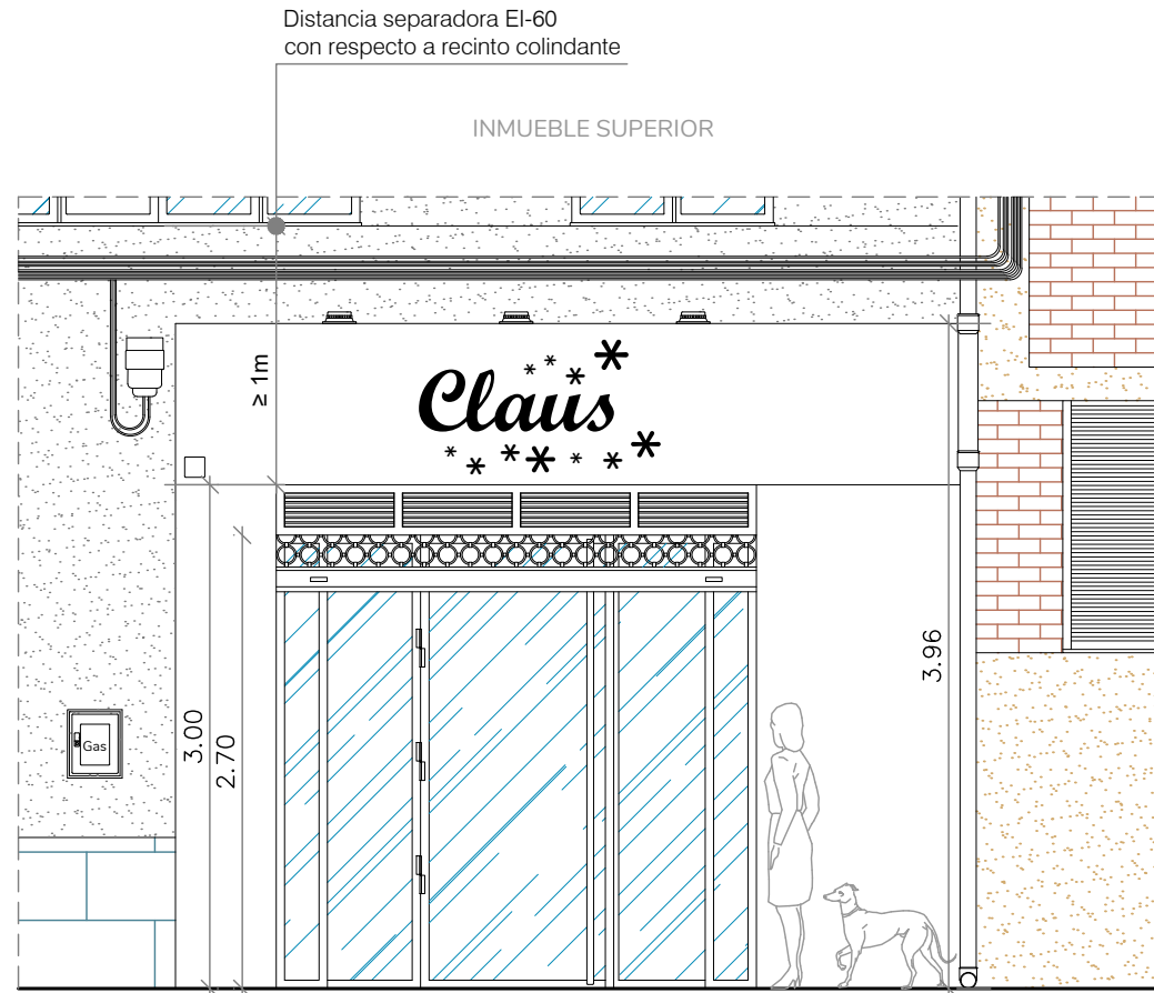
ALZADO EN ESTADO ACTUAL DE FACHADA E:1/50
