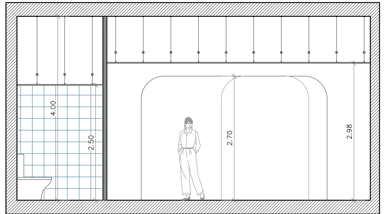
SECCIÓN C-C'
