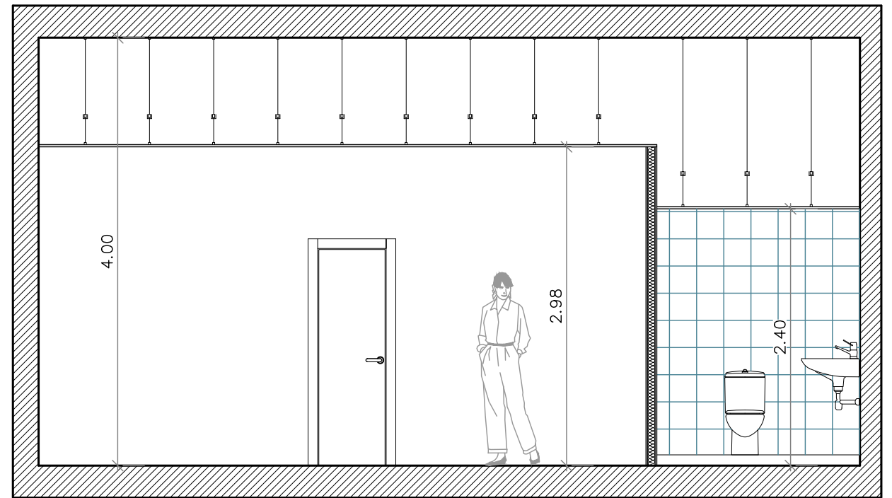
SECCIÓN C-C'
