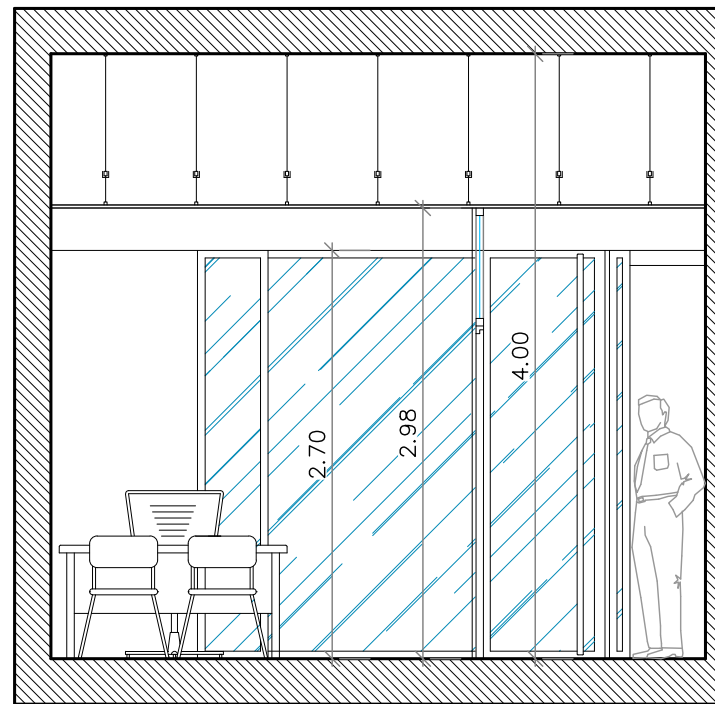
SECCIÓN B-B'
