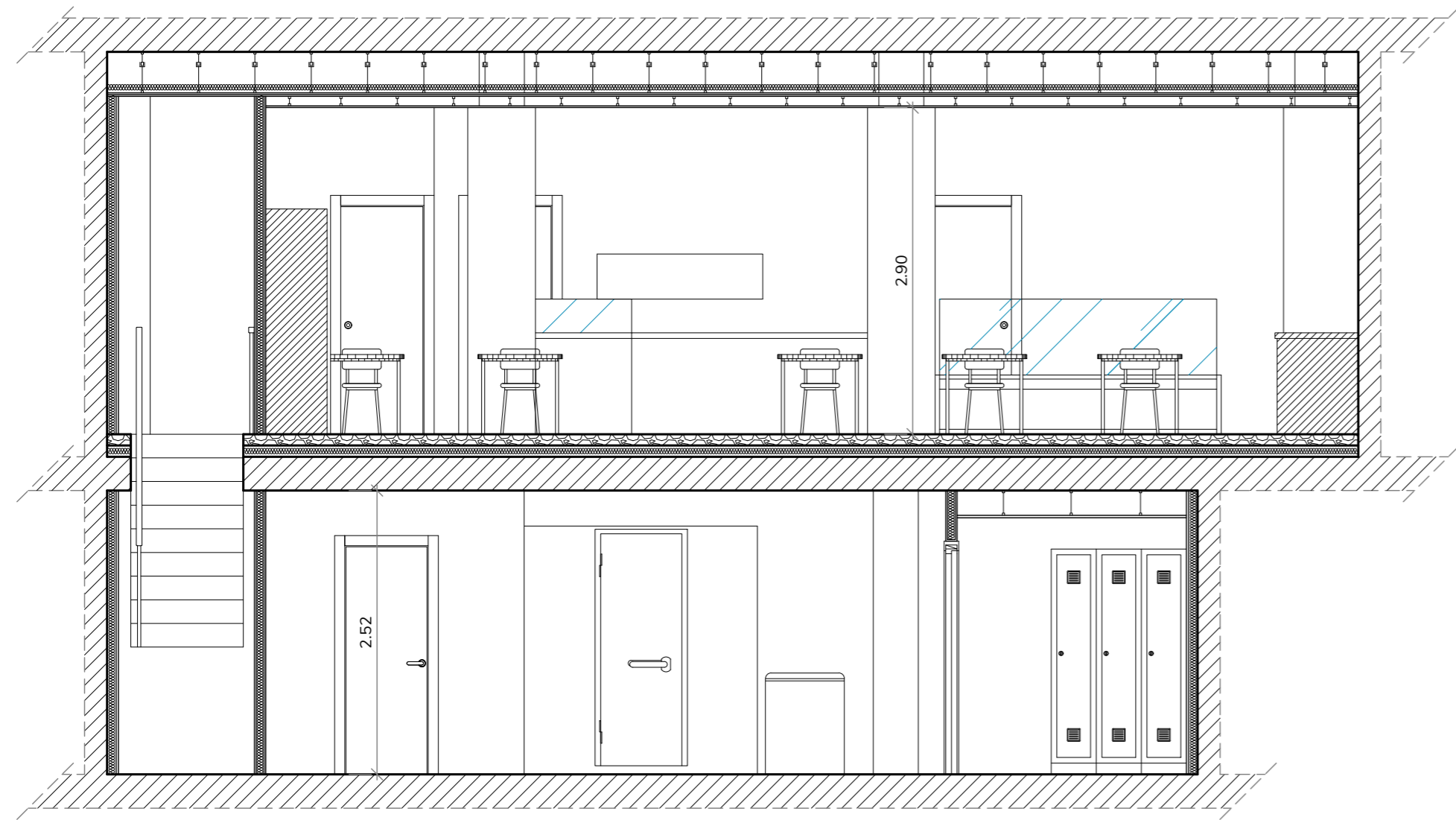
SECCIÓN α-α' EN ESTADO PROPUESTO, E:1/50
