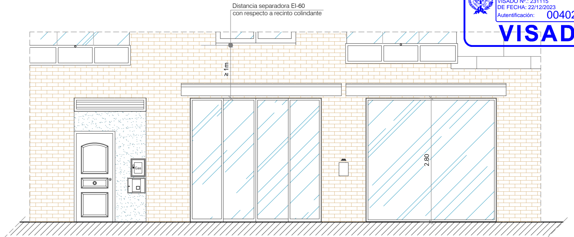
FACHADA EN c/CLAVIJO ESTADO ACTUAL, E:1/50
