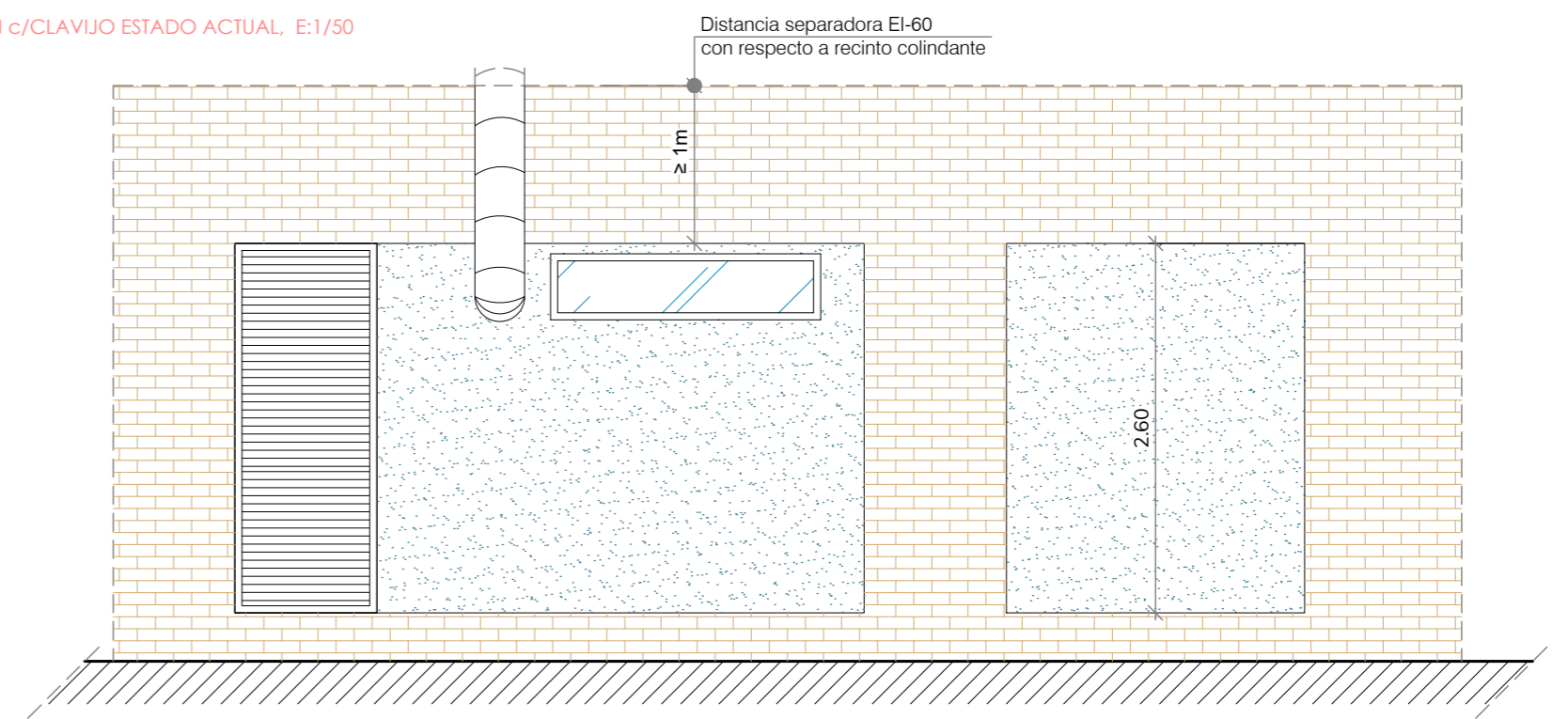
FACHADA POSTERIOR A PATIO EN ESTADO ACTUAL, E:1/50
