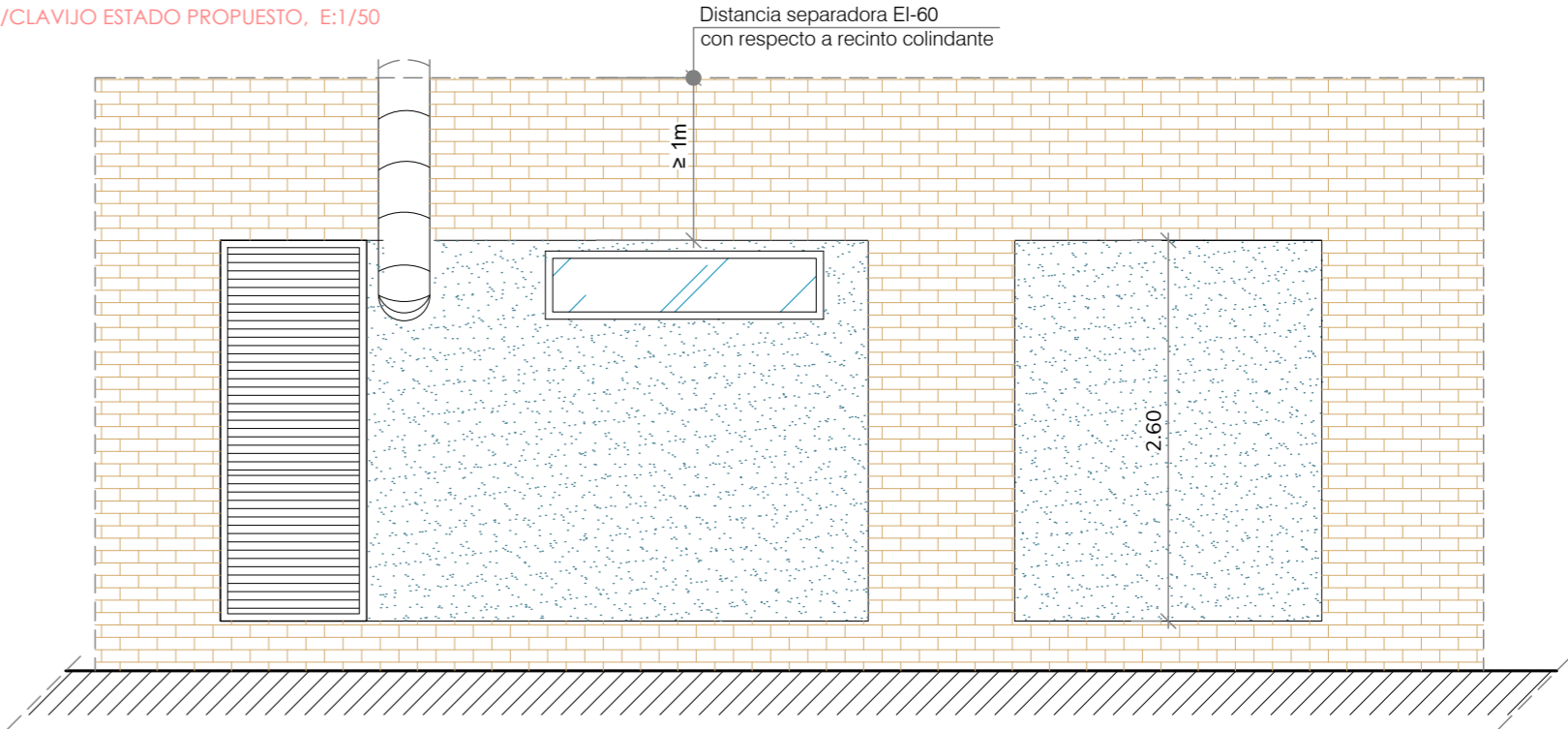
FACHADA POSTERIOR A PATIO EN ESTADO PROPUESTO, E:1/50
