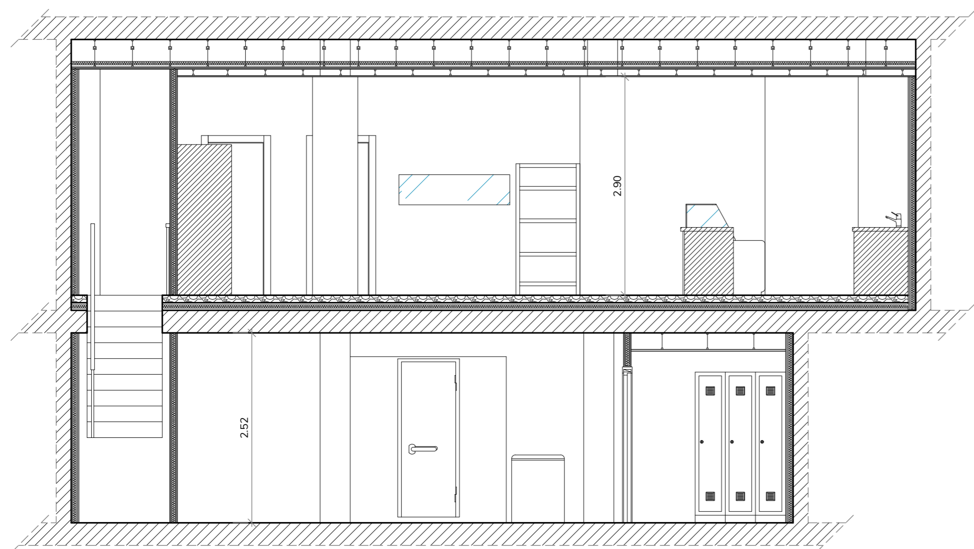
SECCIÓN α-α' EN ESTADO ACTUAL, E:1/50
