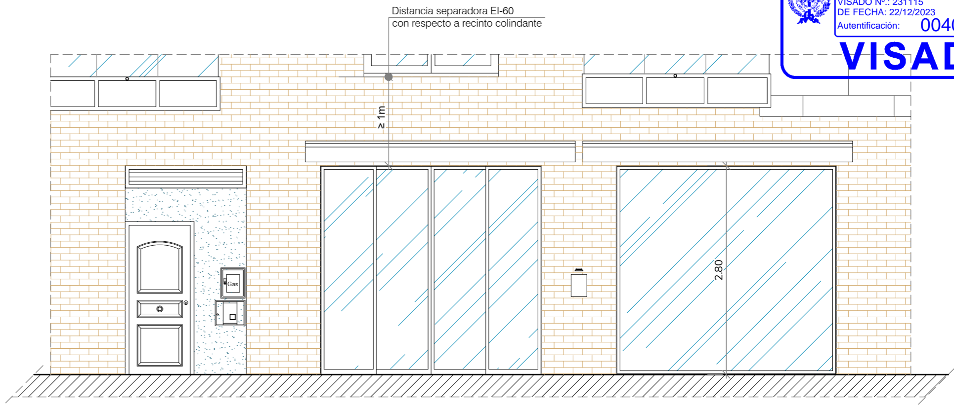
FACHADA EN c/CLAVIJO ESTADO PROPUESTO, E:1/50
