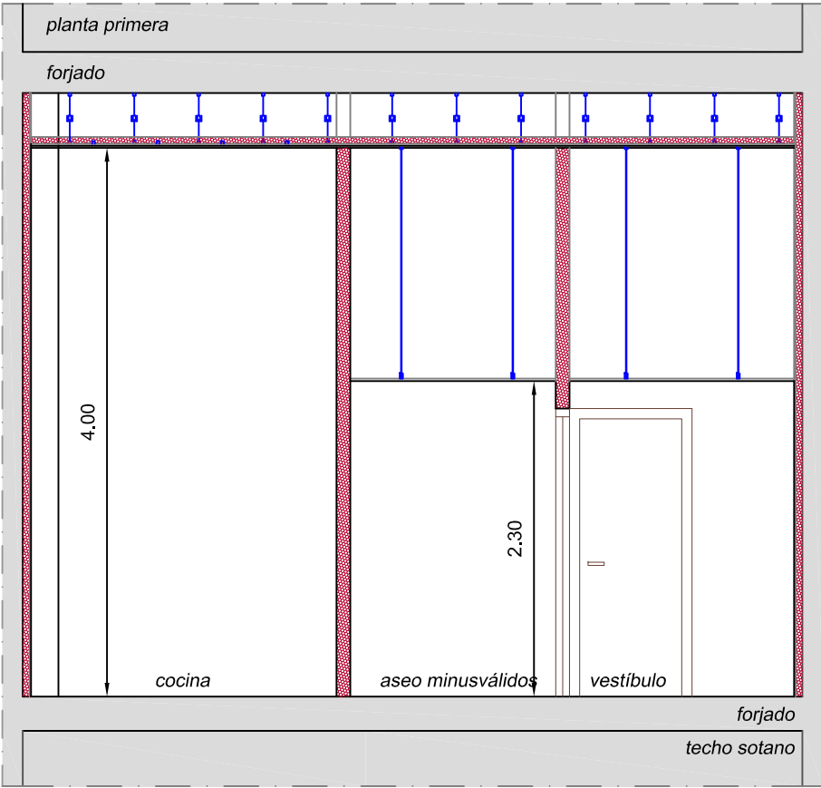
SECCIÓN C - C '
