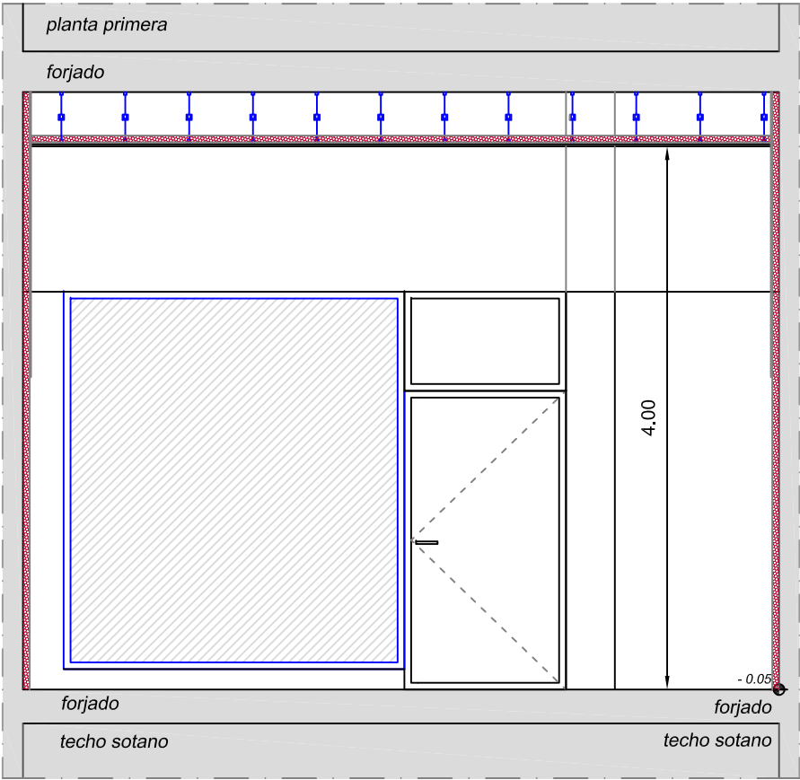
SECCIÓN B - B '
